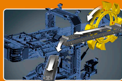
Laufende Förderbänder
